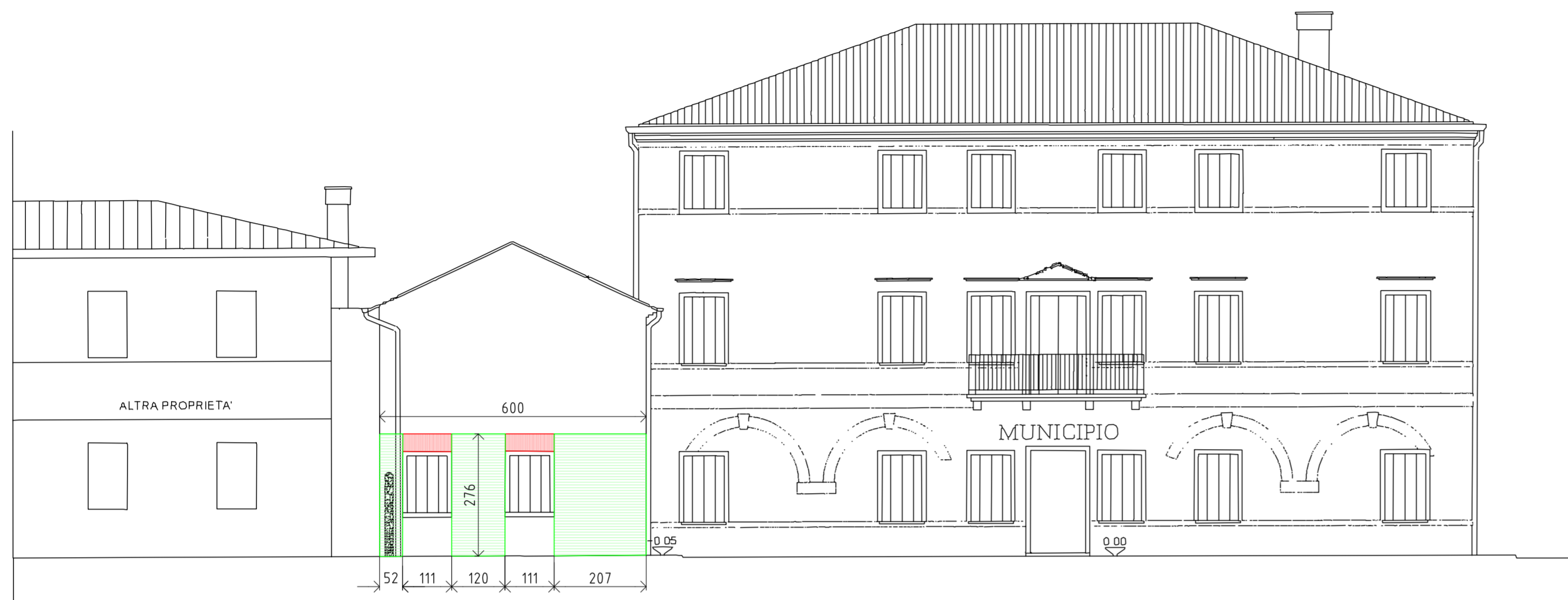
PROSPETTO SUD POVEGLIANO - SEDE COMUNALE
