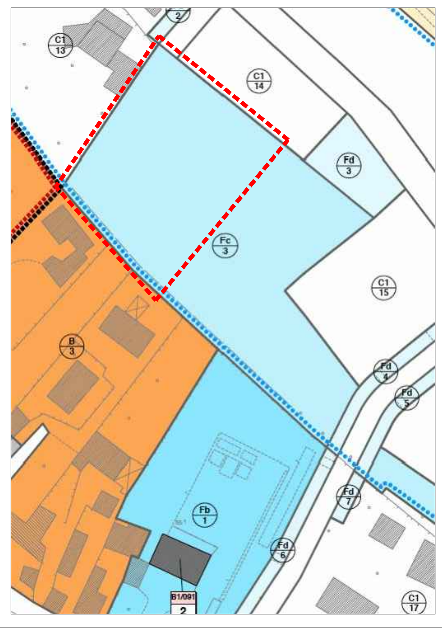
ESTRATTO DI P.I. SCALA 1:1000
