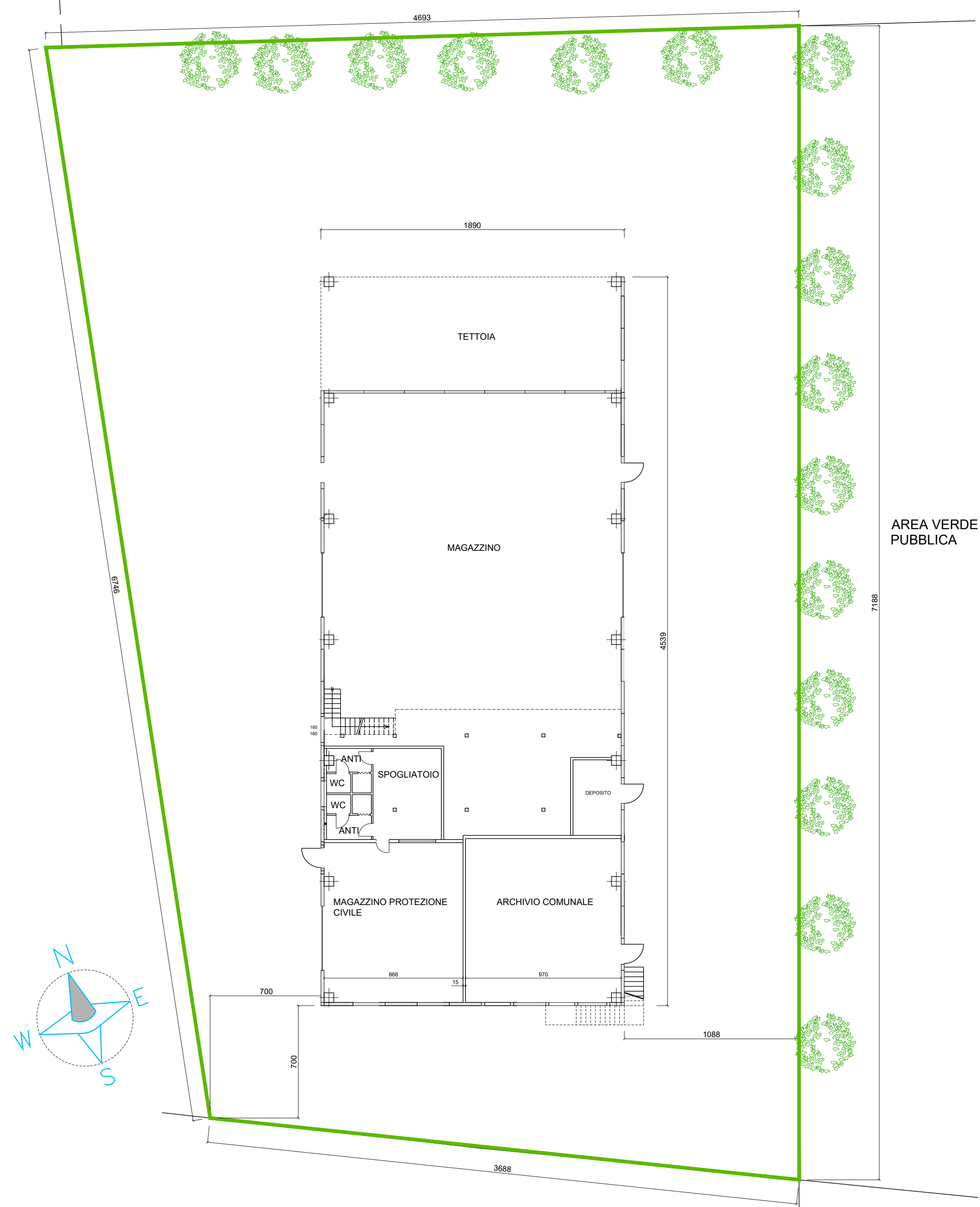
PLANIMETRIA GENERALE Scala 1:200
